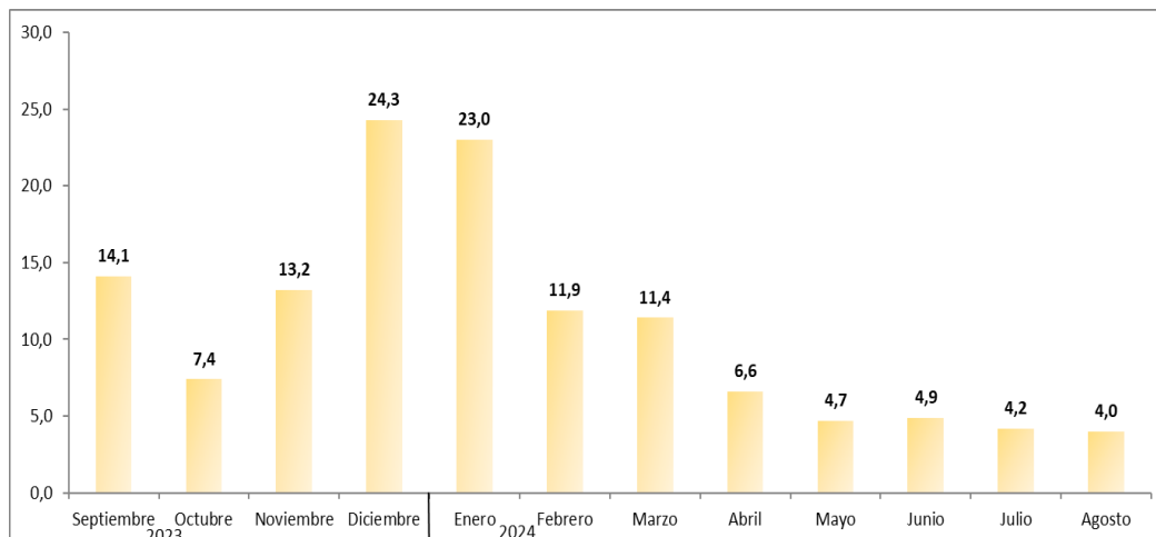
Gráfico N°1. IPCSJ - Variación porcentual mensual. Nivel general. Agosto 2024
