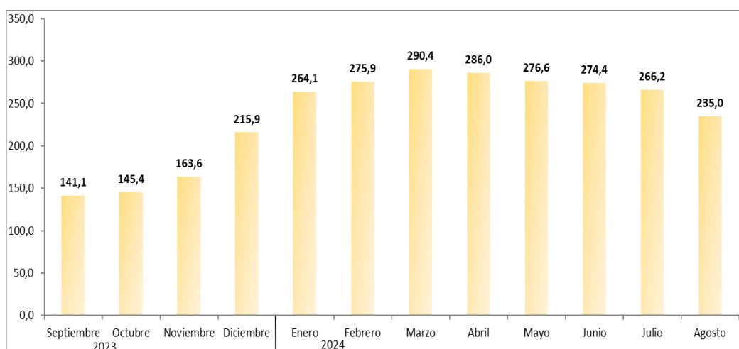
Gráfico N°2. IPCSJ - Variación porcentual interanual. Nivel general. Agosto 2024
